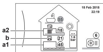
a1 Warmteafgever in de primaire zone (in dit voorbeeld vloerverwarming)
