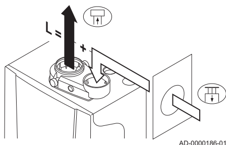
Afb.11 Verschillende drukgebieden
