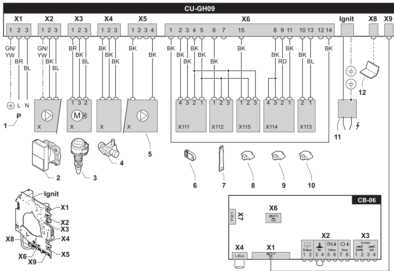
Afb.99 Elektrisch schema
